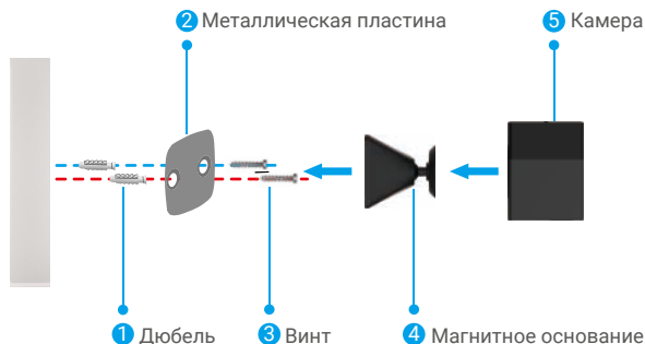
Рисунок 2. Монтаж шурупами
